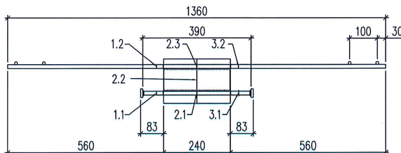
Figure 1 Représentation schématique de l'échantillon d'essai (coupe) (représentation fournie par le donneur d'ordre).
