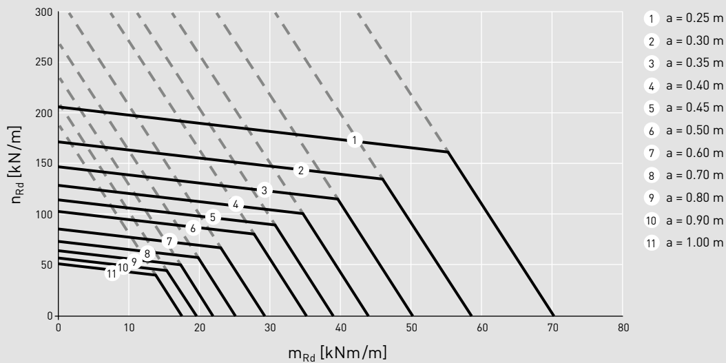
Anwendungsfälle: C Diagramm: C25.1
