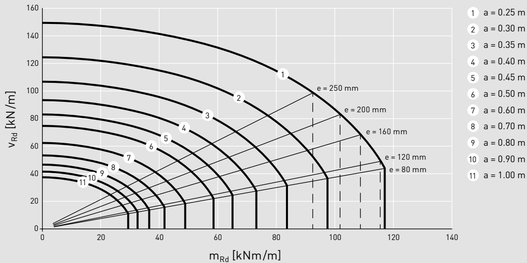
Anwendungsfälle: B Diagramm: B26.3
