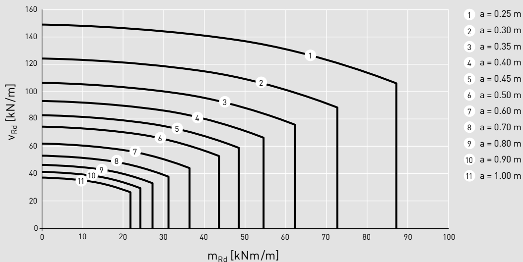
Anwendungsfälle: C Diagramm: C26.3
